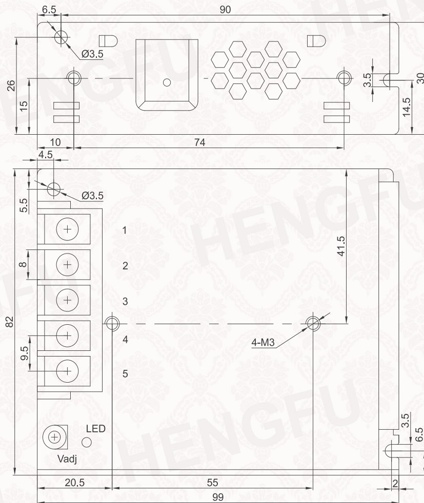
机壳 Frame
